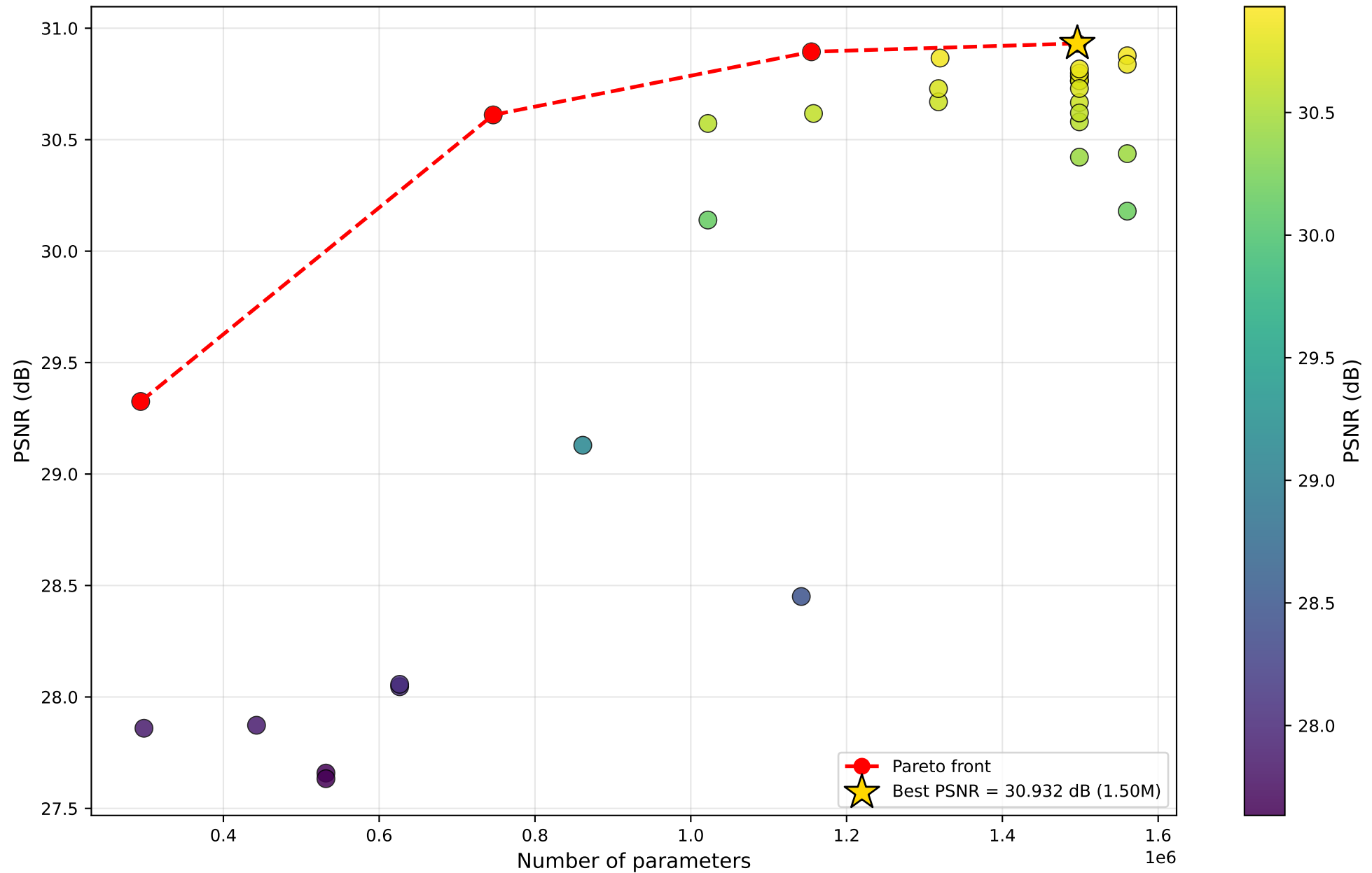
PSNR vs #Parameters — DAT
